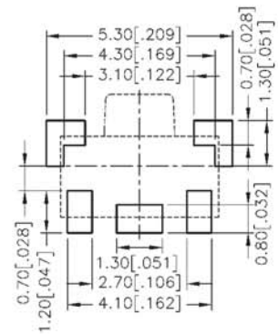
P.C.B. LAYOUT
